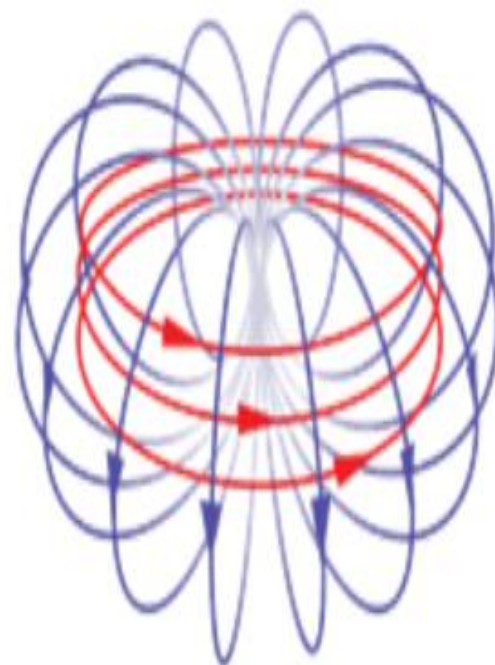
электромагнитное поле
