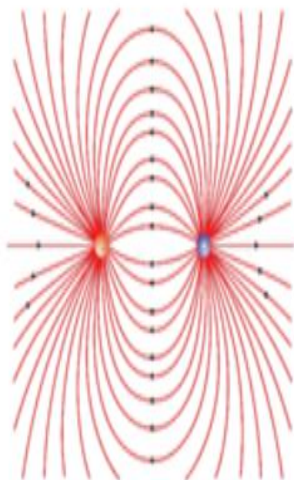
электрическое поле
