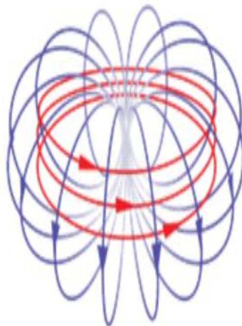
электромагнитное поле
