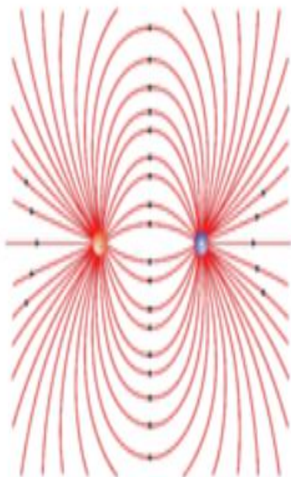
электрическое поле
